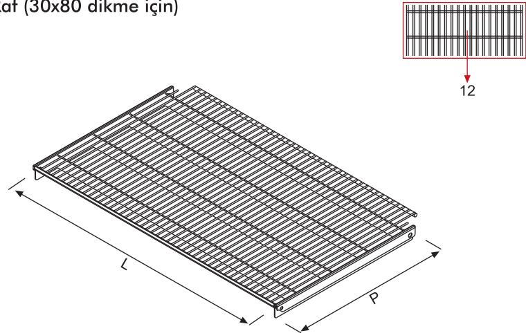
Wire Shelf (for 30x80 upright) Tel Raf (30x80 dikme için)
