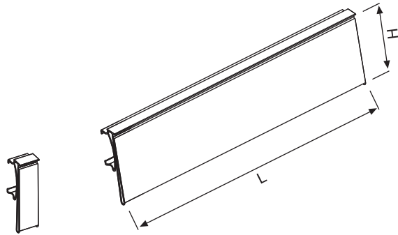
Label Holder External Corner Raf Etiketliği Dış Köşe
