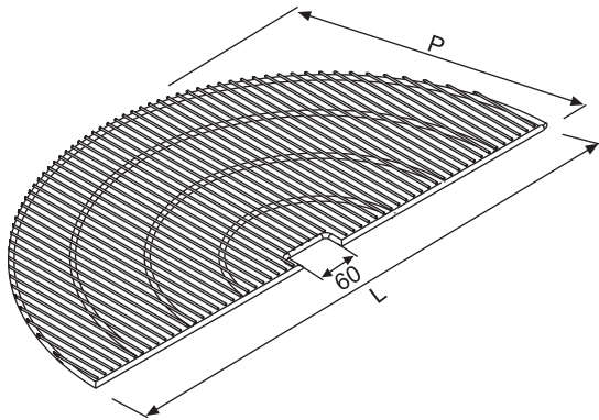
Rounded Wire Shelf (for 30x60 upright) Yuvarlak Gondolbaşı Tel Raf (30x60 dikme için)
