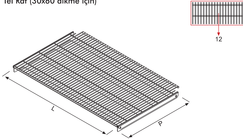
Wire Shelf (for 30x60 upright) Tel Raf (30x60 dikme için)
