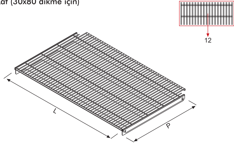
Wire Shelf (for 30x80 upright) Tel Raf (30x80 dikme için)
