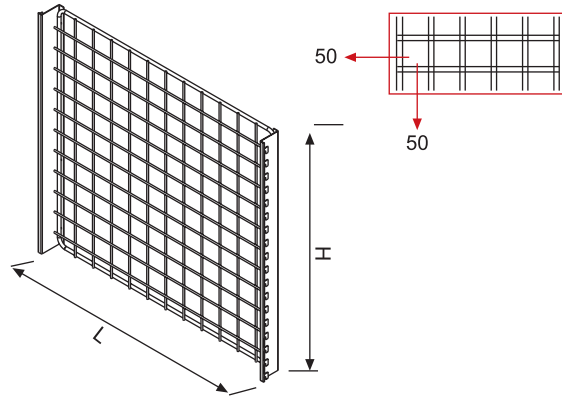
Wire Back Panel (for 30x60 upright) Tel Arka Pano (30x60 dikme için)
