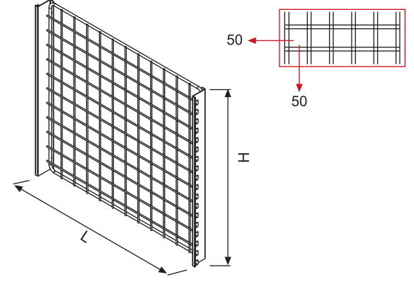
Wire Back Panel (for 30x80 upright) Tel Arka Pano (30x80 dikme için)
