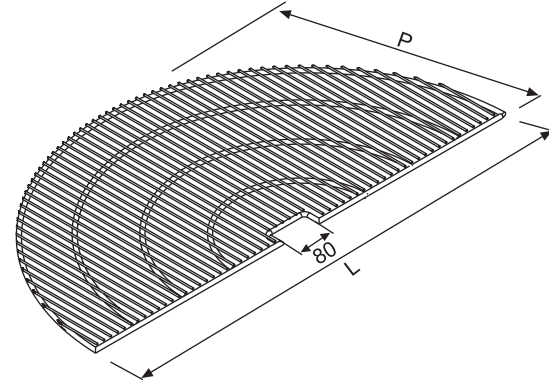
Rounded Wire Shelf (for 30x80 upright) Yuvarlak Gondolbaşı Tel Raf (30x80 dikme için)
