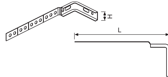
Fixing Part Duvara Bağlantı Aparatı
