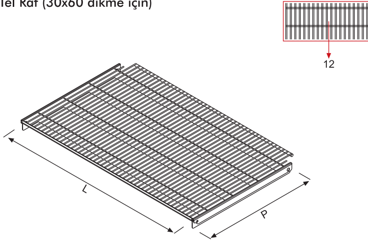
Wire Shelf (for 30x60 upright) Tel Raf (30x60 dikme için)
